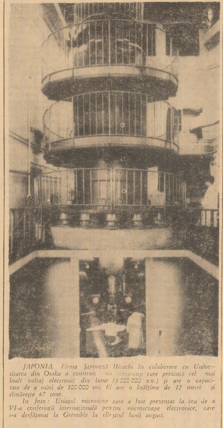
JAPONIA. Firma japoneză Hitachi în colaborare cu Universitatea din Osaka a construit un microscop care prezintă cel mai înalt voltaj electronic din lume (300000 e.v.) și are o capacitate de 600 de milioane de ori. El are o înălțime de 12 metri și cântărește 67 tone.
