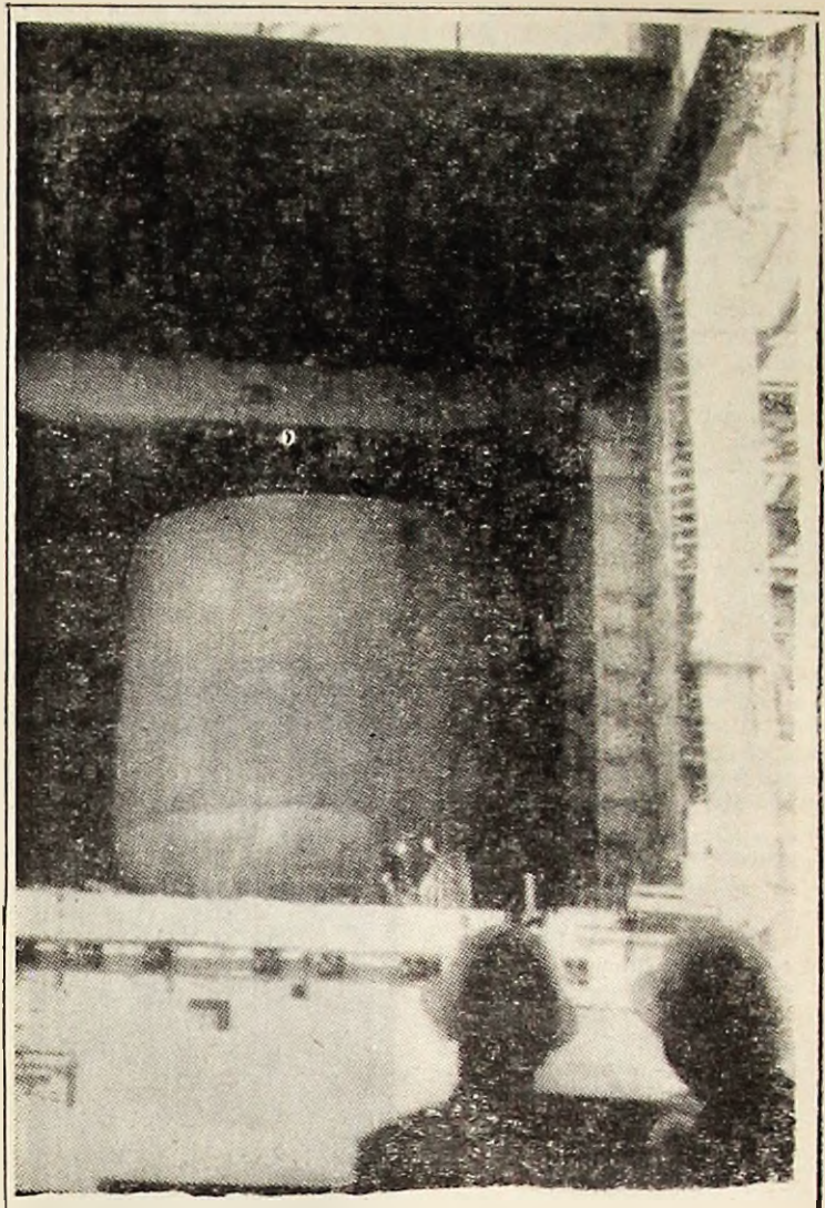
FRANȚA: În 1973 va intra în funcțiune pila de regenerare a neutronilor rapizi de la Phoenix de Miorcau. În foto: Coborârea lentă a cunei de 135 de tone în care va fi instalată inima reactorului. Cupa are o înălțime de 14 m și un diametru tot de 14 m.
