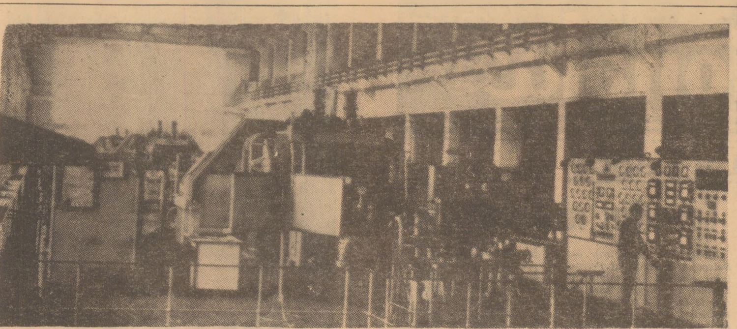
Termocentrala Poroșeni — sala turbinelor
