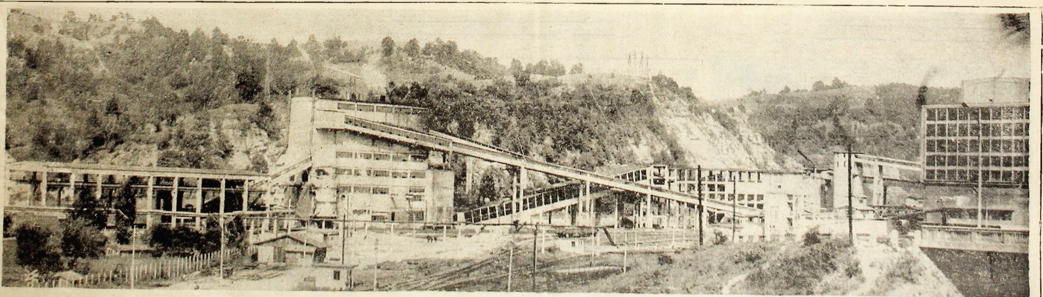
Imagine de ansamblu a fabricii de brichete din Coroești, obiectiv de seamă, realizat în cîincinalul trecut, care ridică pe o treaptă superioară valorificarea cărbunilor extrași din adîncul Văii Jiului
