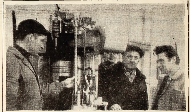
În atelierul-școală de la Depoul C.F.R. Petroșani se învață pe viu funcționarea locomotivelor Diesel. Într-o discuție purtată în atelier pe instructorul Alexandru Hașca, mecanoicul Ion Dascălu, maestrul Aurel Cazan și, în spate, tehnicianul Andrei Despa. Foto: E. FRITSCH
