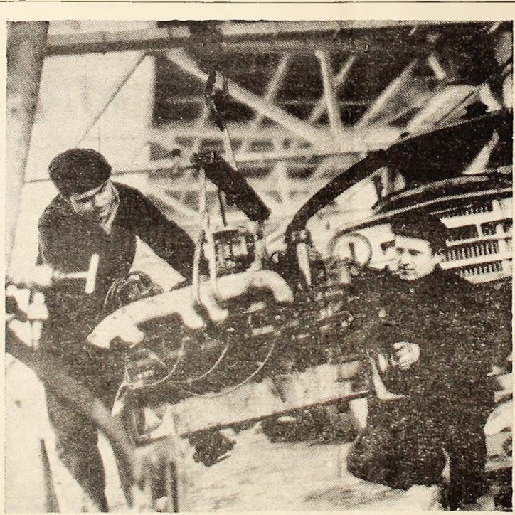
Ilustrativă, privind preocuparea conducerii I.T.A. Autobaza nr. 3 Petroșani pentru introducerea micii mecanizații în procesul de întreținere, este și această macara pentru demonstrație și montarea motoarelor de autovehicule.
