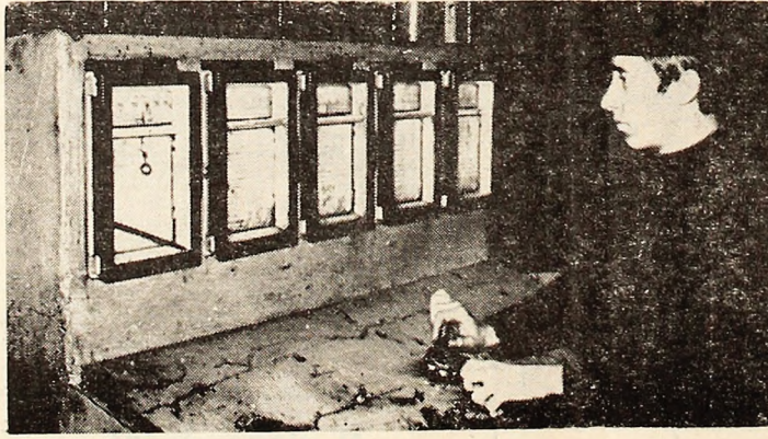
Secția stîlpi hidraulici din cadrul atelierului electro-mecanic al minei Lupeni — aparatul de înregistrare a presiunii.
