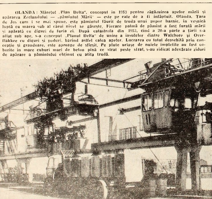
În foto: Partea de sud a digului este construită din blocuri de beton, partea de nord din chesoane. Aici partea de nord a digului.
