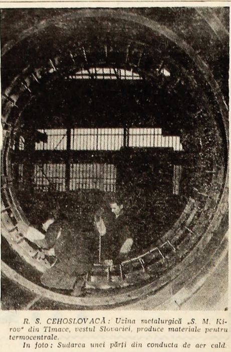
R. S. CEHOSLOVACĂ: Uzina metalurgică „S. M. Kirov” din Timce, vestul Slovaciei, produce materiale pentru termocentrale. În foto: Sudarea unei părți din conducta de aer cald.
