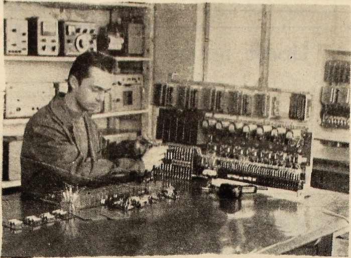
In laboratorul de mecanizare-automatizare, insinerii cercetător Alexandru Albu verifică o instalație de automatizare pentru subteran proiectată și executată de I.C.P.M.H.
