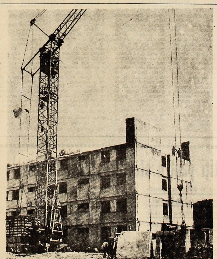
La construcția blocurilor de locuințe de pe șantierul I Petroșani (Aeropot) al T.C.H. se aplică cu bune rezultate metoda de execuție cu panouri mari din prefabricate de beton. Foto: I. LICIU
