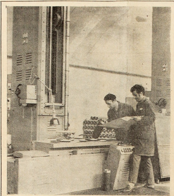
La mașina de homit, cu care a fost de curind utilitată Fabrica de stâlpi hidraulici din Vulcan, maistrul șef Mihai Gudaș și șeful C.T.C. Ion Filip au fost imortalizați pe peliculă verificind calitatea și rugozitatea suprafeței interioare a cilindrilor pentru stâlpi S.V.J.-80. De amintit că rugozitatea este de ordinul... micronilor. Foto I. LICIU
