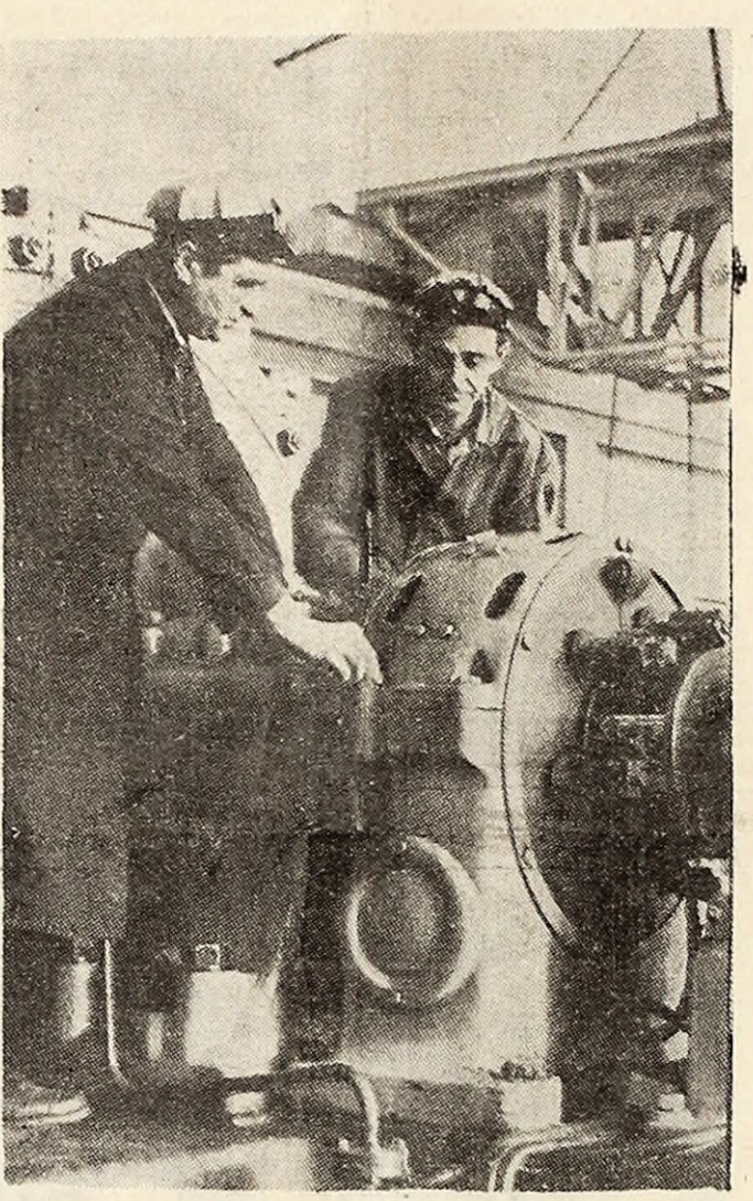
Maiștrii Nicolae Bendea și Vasile Haiduc surprinși de obiectivul aparatului în timp ce verificau excitatoarea generatorului nr. 2 de la Centrala electrică Vulcan. Foto I. LICIU
