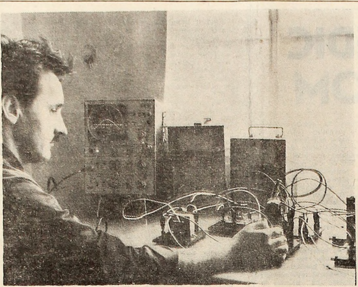
O nouitate la U.U.M.P.: Atelierul de automatizare care produce echipament electric pentru industria minieră. În clădire, inginerul Alexandru Scroban la standul pentru verificarea și reglarea circuitelor electronice făcînd o verificare a acestor parametri cu ajutorul osciloscopului. Foto: I. LICIU
