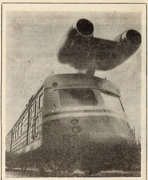
U.R.S.S. Rapidul din Kalinin. Vagonul rapid — laborator cu tracțiune reactivă — a fost construit la Uzina constructoare de vagoane din Kalinin. Viteza lui atinge 250 km/oră. E folosit pentru cercetări aerodinamice și în legătură cu construcția de trenuri expres de mare viteză.
