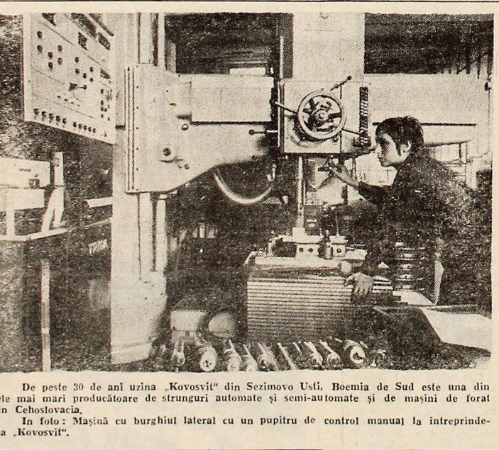
De peste 30 de ani uzina „Kovosvit” din Sezimovo Usti, Boemia de Sud este una din cele mai mari producătoare de strunguri automate și semi-automate și de mașini de forat din Cehoslovacia. In foto: Mașină cu burghiul lateral cu un pupîtur de control manual la întreprinderea „Kovosvit”.
