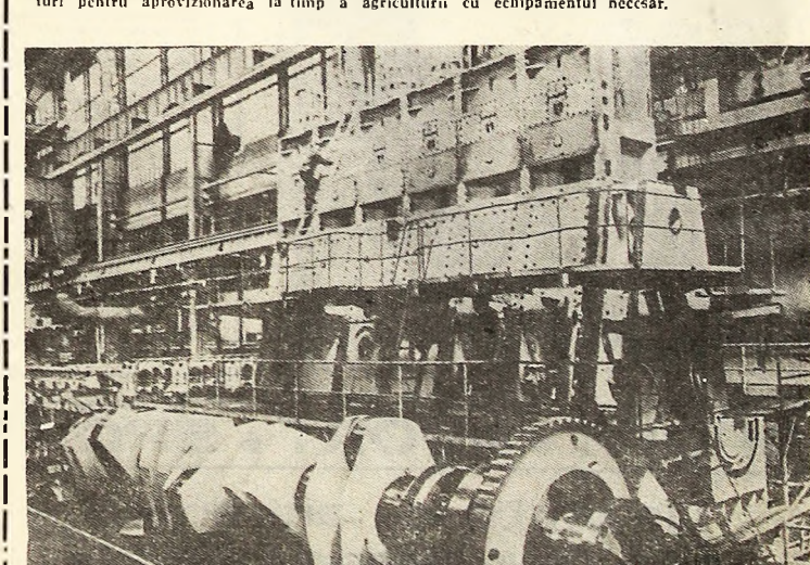
R. P. POLONA: Uzinele din Poznan sînt cea mai importantă producătoare de motoare navale din Polonia. Recent aici a început construcția motorului RDN-76.
