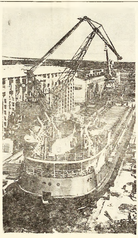
U.R.S.S.: La Șantierea navală Kama din Perm (Ural) se construiește primul vas petrolier oceanic. Lungimea vasului — 120 m, lățimea — 13 m, viteza — 20 km/h. Capacitatea lui este de 1.800 tone încărcătură și 2.700 tone petrol.
