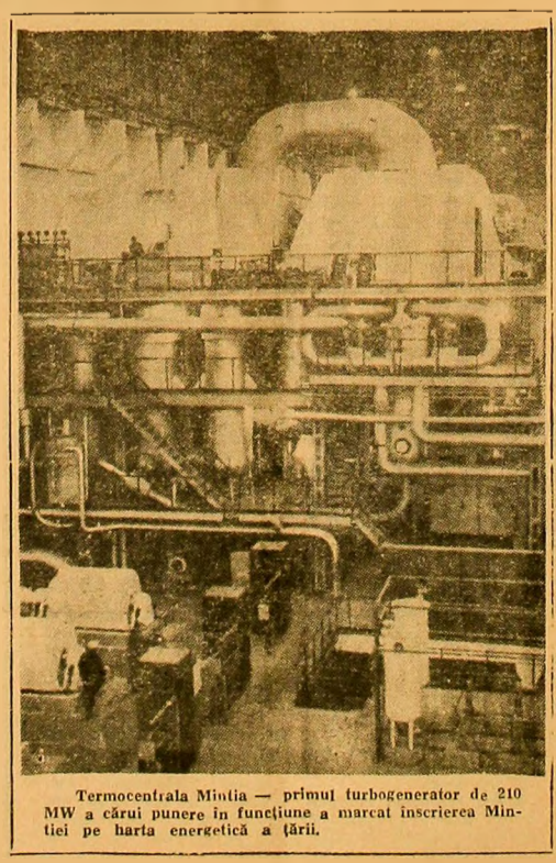
Termocentrala Mintia — primul turbogenerator de 210 MW a căruia punere în funcțiune a marcat înscrierea Mintiei pe harta energetică a țării.
