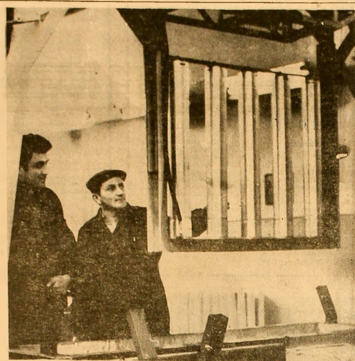
Stilpii hidraulici executați la F.S.H. Vulcan au devenit un echipament indispensabil în tehnologia susținerii abatajelor. Aceștia sînt unul din factorii esențiali în creșterea productivității muncii, reducerea consumului de material lemnos, ușurarea efortului fizic și asigurarea securității muncii în subteran.
