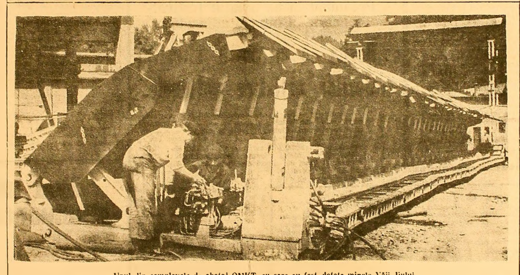
Unul din complexe de abataj OMKT, cu care au fost dotate minele Văii Jiului
