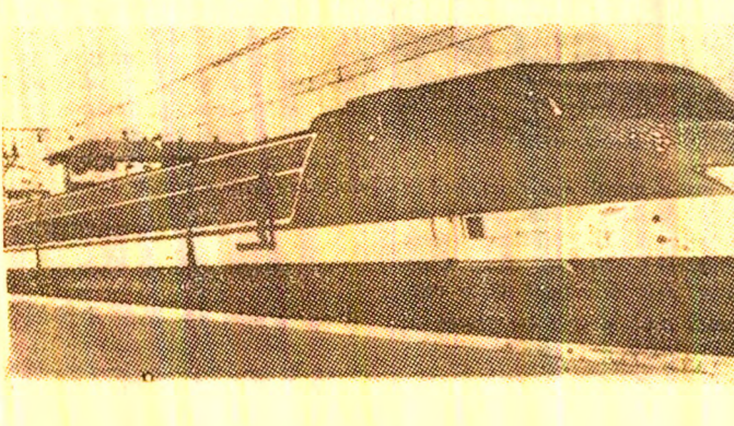
FRANȚA: Turbotrenul experimental de mare viteză TGV COI prezentat la uzinele Alstom din Belfort. Trenul cu acea o viteză de 300 km/h și este echipat cu 4 turbine de 3.720 kW. Testele de mare viteză se vor desfășura în primăvara acestui an în Alsacia.
