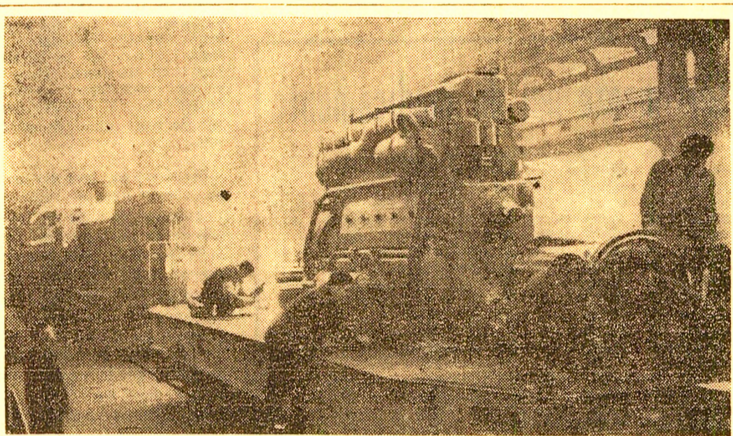
Uzinele „23 August” București, pregătesc pentru anul 1973, locomotive electrice „Diesel” de 1250-1500 C.P. În foto: Montarea unei locomotive de 1250 C.P.
