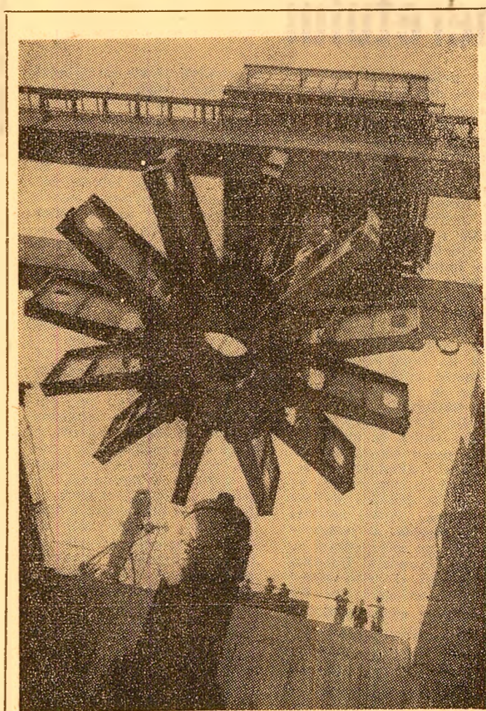
U.R.S.S. În foto: Aspect din timpul lucrărilor de montaj la primul hidroagregat de la hidrocentrala Nurek.
