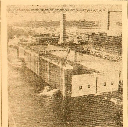
FRANȚA. La Brest urmează să fie dat la apă primul element mare al viitorului bazin nr. 10 destinat submarinelor nucleare. Bazinul cîntărește 17 000 de tone și este fabricat din beton precomprimat. Lungimea sa (totală) va fi de 167 m, lățimea de 30 m și profunzimea de 21 m.
