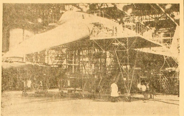
U.R.S.S. — La Uzina constructoare de avioane din Voronej a intrat în producție de serie avionul supersonic de pasageri „TU-144”. În foto: Aspect din hala de montaj a uzinei din Voronej.
