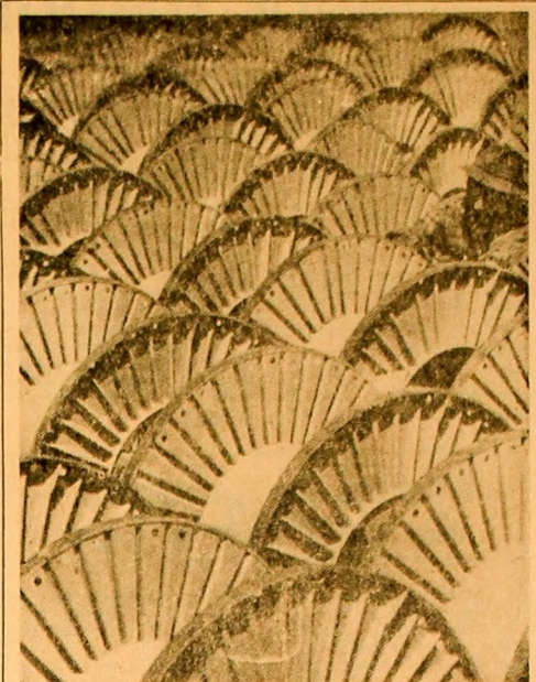
R.P. UNGARA — Compania de industrie metalică din tinutul Nograd produce cabine de tractoare și de basculant, tamburi etc. pentru necesitățile interne și export. În foto: O serie de tamburi gata pentru livrare în curtea fabricii.
