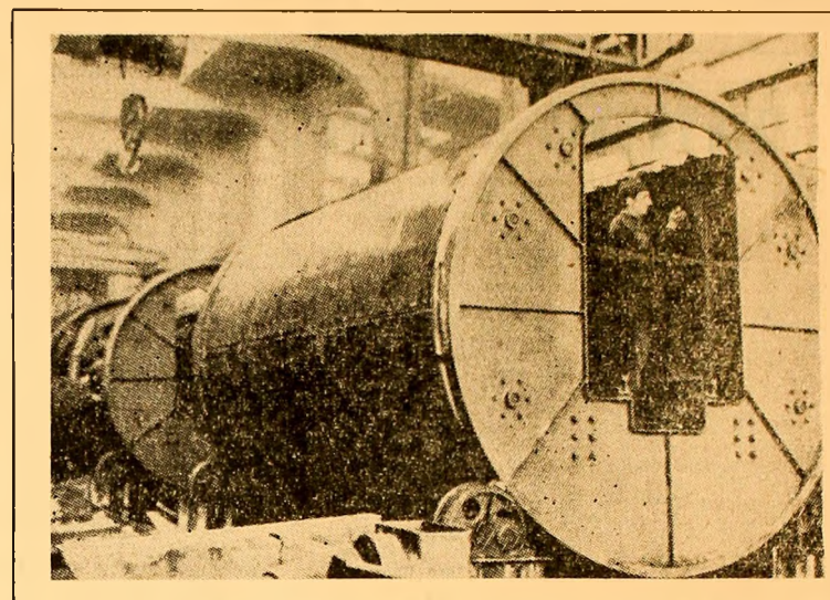
R.P. BULGARIA. Uzina constructoare de mașini „Struma” din Pernik produce mașini pentru industria minieră, dintre care o mare parte este destinată exportului. În FOTO: Mașini de tipul „mașini rotative universale” produse pentru prima dată la această uzină.
