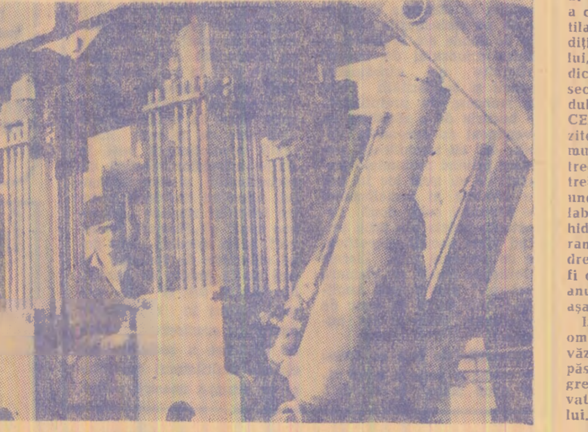
Lăcătușii Ion Petcu, Adalbert Pall și Ion Stancu din brigada de montaj a cadrelor pășitoare condusă de comunistul Iuliu Kocsek, în timpul finalizării montajului unui cadru pășitor.
