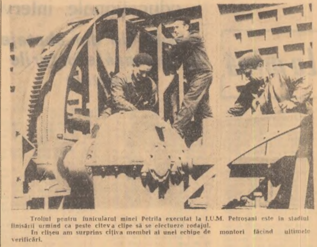
Trolul pentru funicularul minei Petrița executat la I.U.M. Petrosani este în stadiul înisării urmind ca peste cîteva zile să se efectueze rodajul. În clișeu am surprins cîteva membri ai unei echipe de montori făcînd ultimele verificări.
