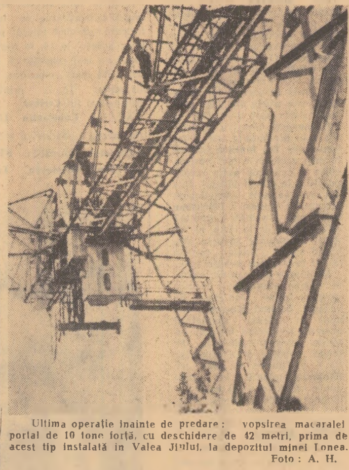
Ultima operație înainte de predare: vopsirea macaralei portal de 10 tone forță, cu deschidere de 42 metri, prima de acest tip instalată în Valea Jiului, la depozitul minei Lonea. Foto: A. H.
