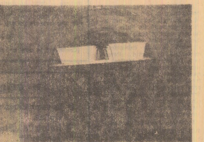
Chișeuș nr. 1 Vase din polistiren expandat umplute cu apă și așezate polite în formale de baraj de oprire a exploziilor din mine.
