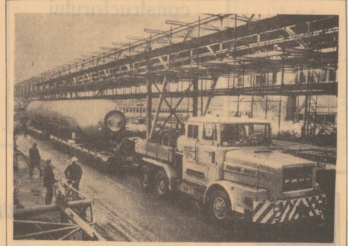
La Combinatul de azot din Piesteritz, R.D.G., a sosit unul din cele trei reactoare cu urae fabricate în Cehoslovacia. El cîntărește aproximativ 210 tone.
