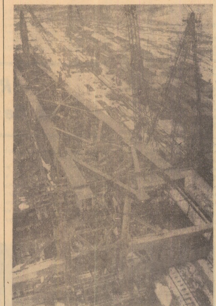
R. D. GERMANA: Imagine din timpul instalării, la mina de lignit din Hagenwerder, a celei mai mari bene de excavator din Europa. Acest gigant se sprijină pe 256 de roți și are o capacitate de 7 800 m³/h.
