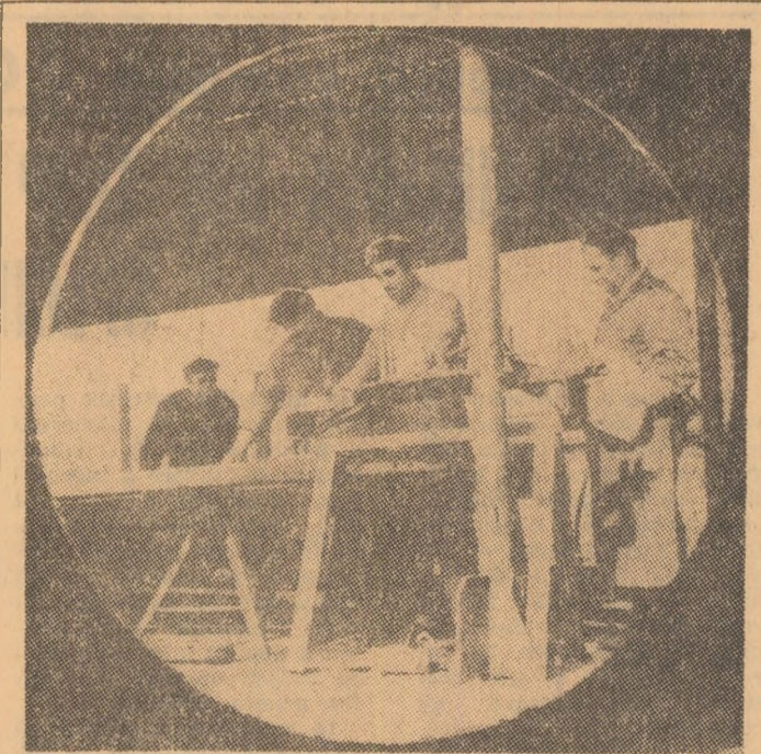
La confecționarea moazetelor cu care va fi armat noul put nr. 11 de la mina Lonea 1-am surprins pe șeful echipei de la confecții metalice a atelierului electromecanic al minii, Ioan Madarasz împreună cu colegii de echipă în plină activitate.
