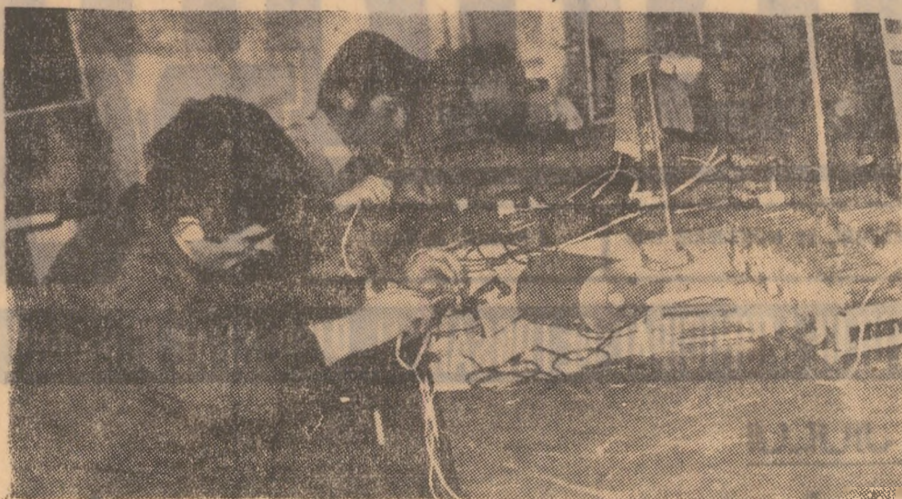
Studentii V. Cernăianu și N. Giurgulescu executind o lucrare în laboratorul de automatizări.
