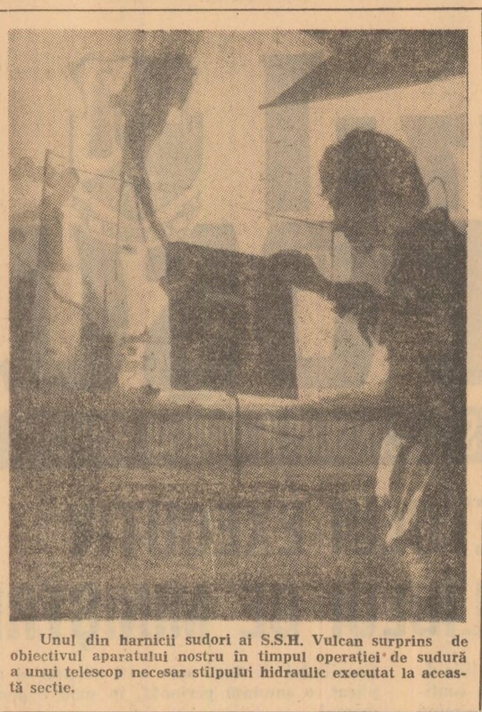
Unul din harnicii sudori ai S.S.H. Vulcan surprins de obiectivul aparatului nostru în timpul operației de sudură a unui telescop necesar stîlpului hidraulic executat la această secție.
