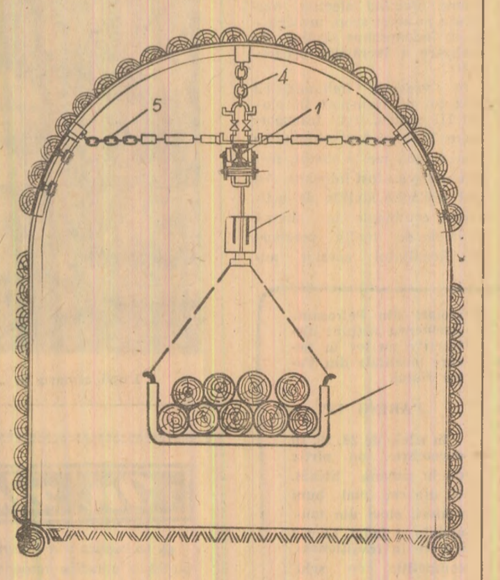
Principalele părți componente ale monoraiului: 1. Cablu de rulare; 2. Cărucior; 3. Platformă; 4. Dispozitiv de suspendare vertical; 5. Suport de ancorare lateral.
