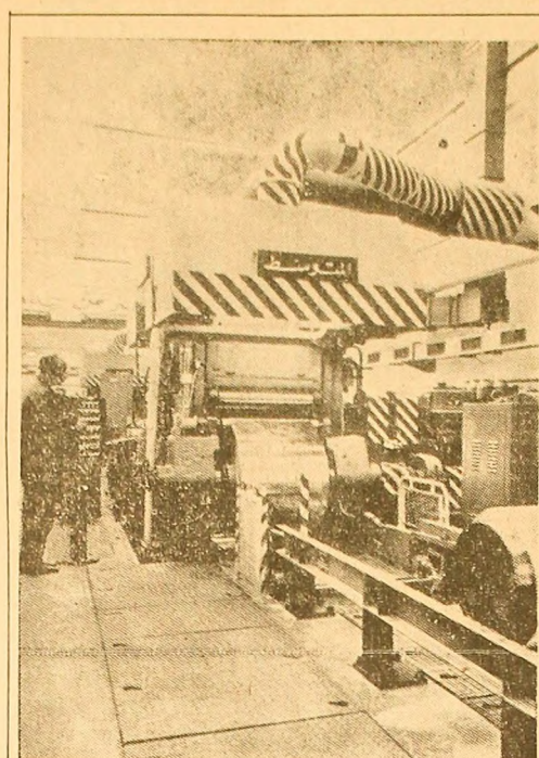
Vedere parțială a laminorului de tablă subțire din Allexandria (R. A. Egipt) care va atinge în final o capacitate de producție anuală de 1.000 tone de tablă de aluminiu.
