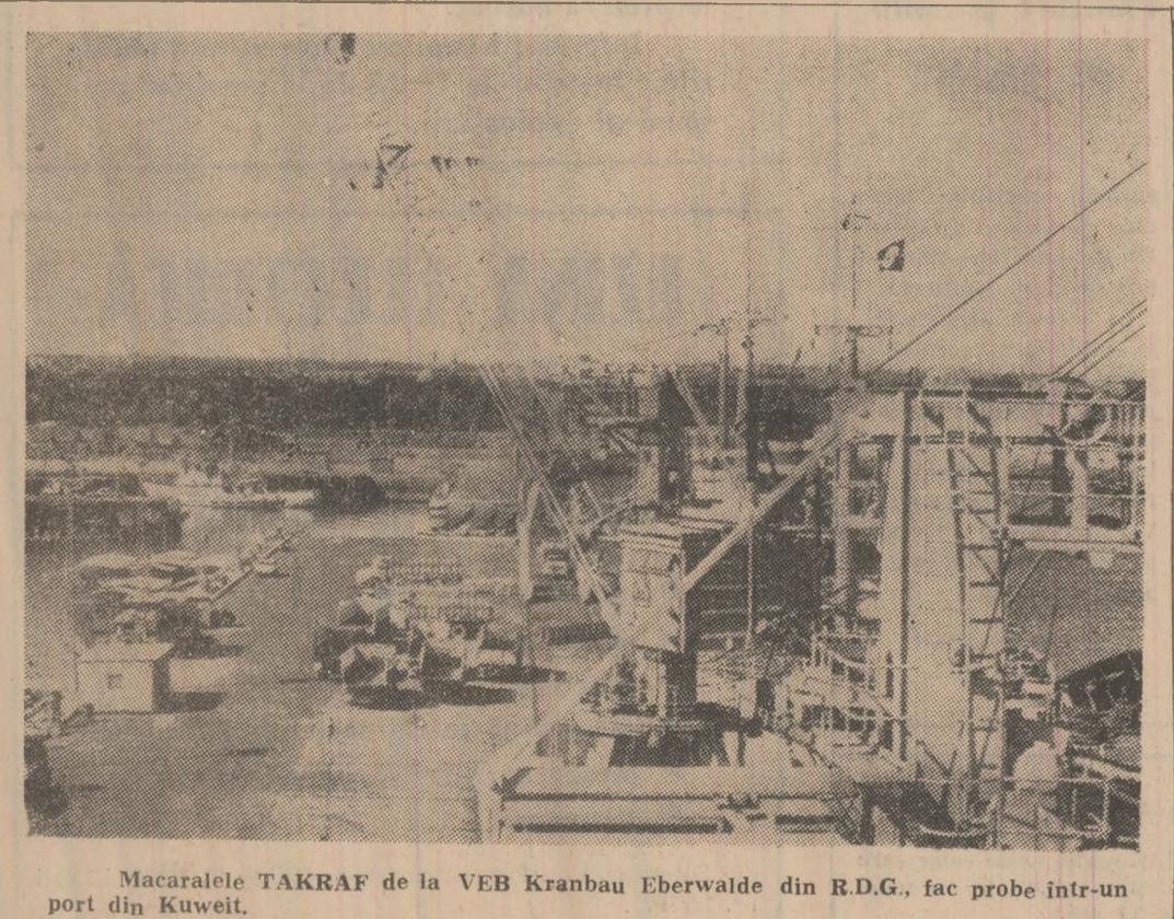
Macaralele TAKRAF de la VEB Kranbau Eberwalde din R.D.G., fac probe într-un port din Kuweit.
