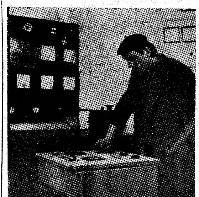
La standul de probe, de la atelierul electric al minei Livezeni, șeful de echipă Gheorghe Dobre încearcă rezistența de străpungere a unui motor.
