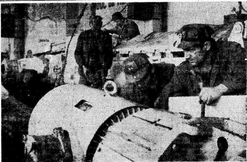
Echipa condusă de lăcătușul Iosif Nagy, din cadrul formației „service” a sectorului V electromecanic al minei Paroșeni, montează transportorul unui nou complex în vederea probelor de atelier. Foto: Ion LICIU
