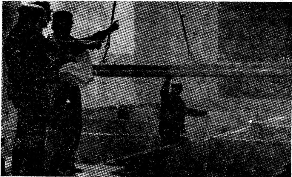
Echipele de montori conduse de Mihai Boboi a trecut la montarea planșelor ultimului etaj al noului bloc 8 de pe strada V. Roaită din Petroșani.
