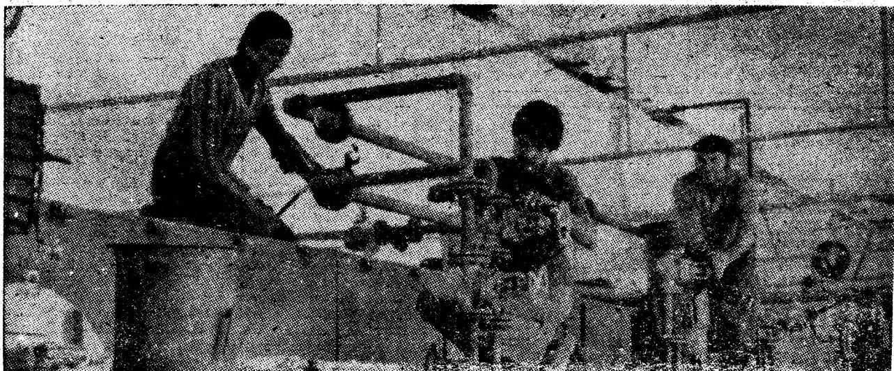
La Fabrica de mobilă se fac reglările instalației la tunelul de uscare din secția finisaj.
