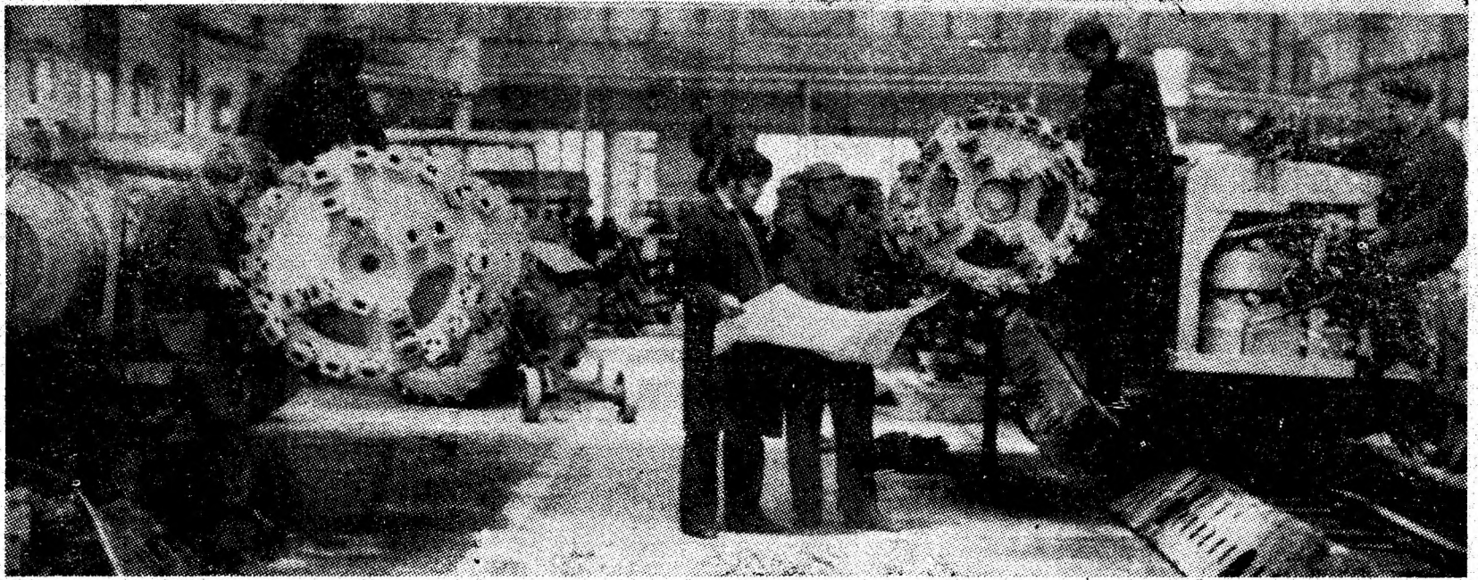
Echipa de lăcătuși condusă de Aurel Lăban finalizează lucrările de montaj a două combine CA-1, ce urmează a fi expediate unor întreprinderi miniere din țară. Foto: Șt. NEMECSEK
