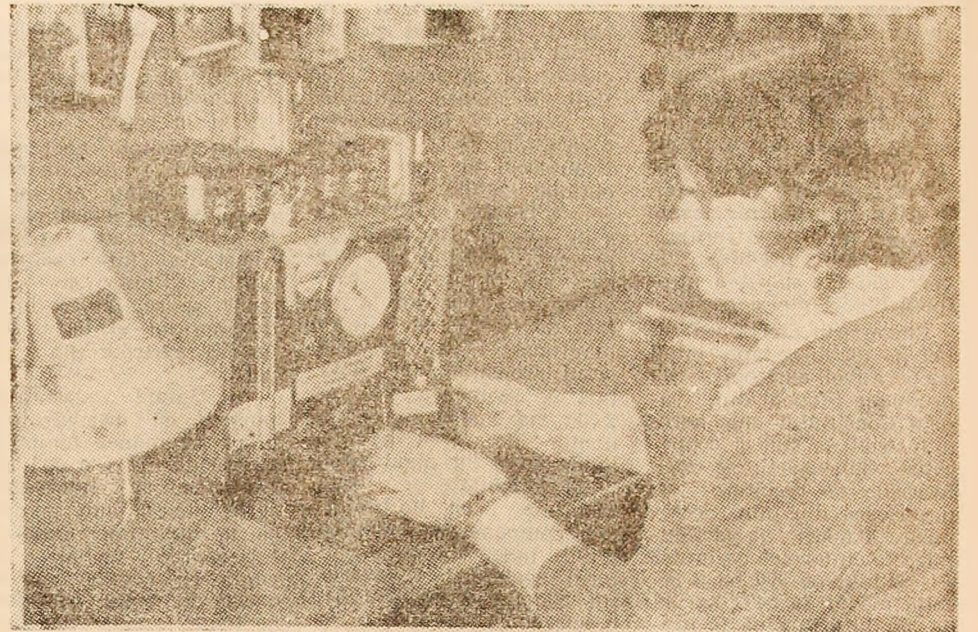
Pentru verificarea concentrațiilor de metan din minele din Vale sunt utilizate detectoare moderne de metan cu precizii mari de măsurare. Ele sunt întreținute și exploatate de personal bine pregătit profesional pentru a asigura securitatea muncii în subteran. În clișeu: muncitorul Viorica Pavel de la laboratorul „Metanometre” al I.M. Vulcan în timpul reglării unui lot de metanometre. Foto: Ioan BĂLOI
