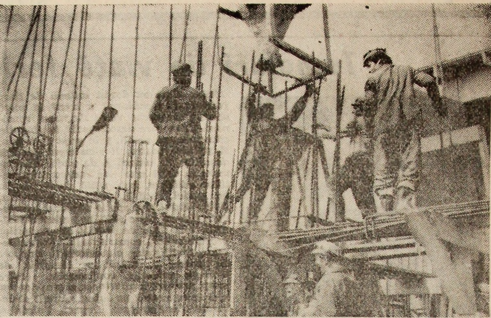
Echipe de betonisti condusa de Mihai Dumitru de pe santierul de constructii al putului cu schip de la I.M. Lupeni, pregatesc turnarea betoanelor in cofrajele cu armatura metalica in diafragme, la cota 29 m.
