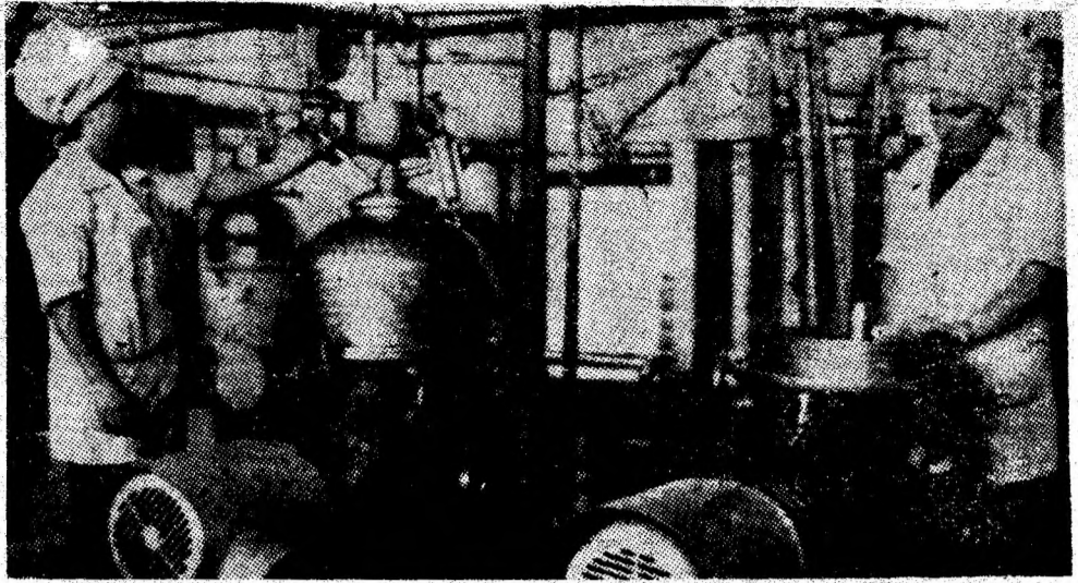
Muncitoarele Săftica Darie și Georgeta Bucicioiu, reglează parametrii de funcționare a instalației de pasteurizare a laptei de la Fabrica de lapte Livezeni.
