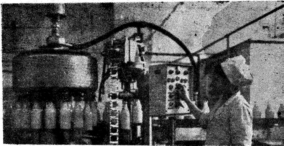
Fabrica de produse lactate. La sectorul de îmbutelire a laptei, instalațiile automatizate sînt servite de un personal muncitor cu pregătire adecvată.
