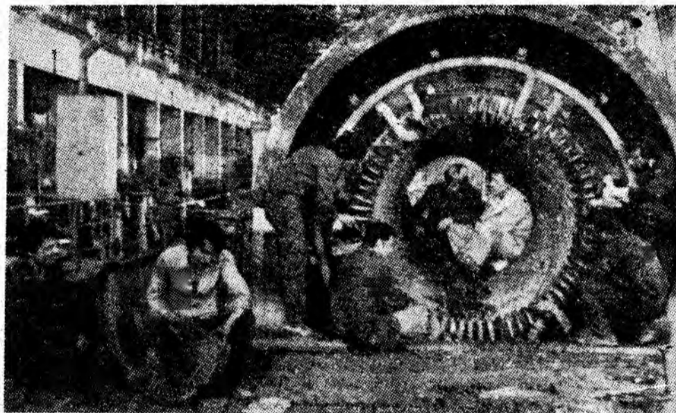
Uzina electrică Paroșeni. Echipa condusă de Nicolae Santi efectuează modificarea turbogeneratorului nr. 1, în vederea conectării la sistemul de termoficare. Foto: Șt. NEMECSEK
